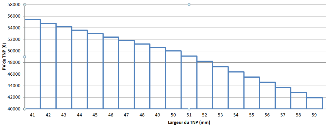
Courbe d'incitation du PV en fonction de la largeur
