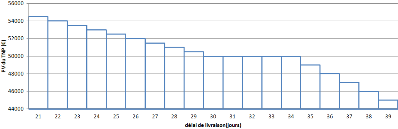
Courbe d'incitation du PV en fonction du délai
