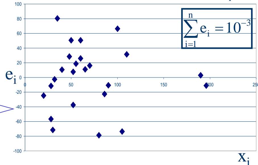
Ecarts résiduels en fonction de x_i
