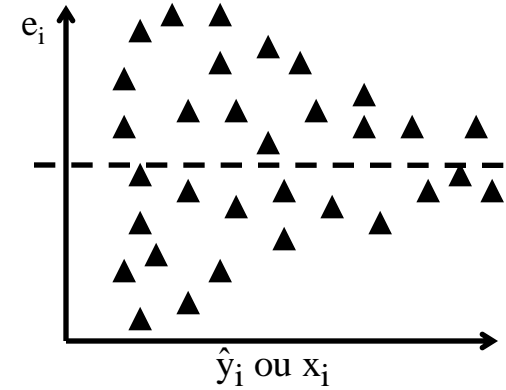
\hat{y}_i ou x_i Variance non constante (petites valeurs de y )
