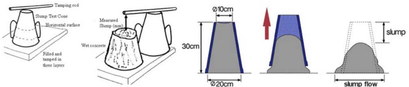
FIGURE 1 – Test de qualité du béton
