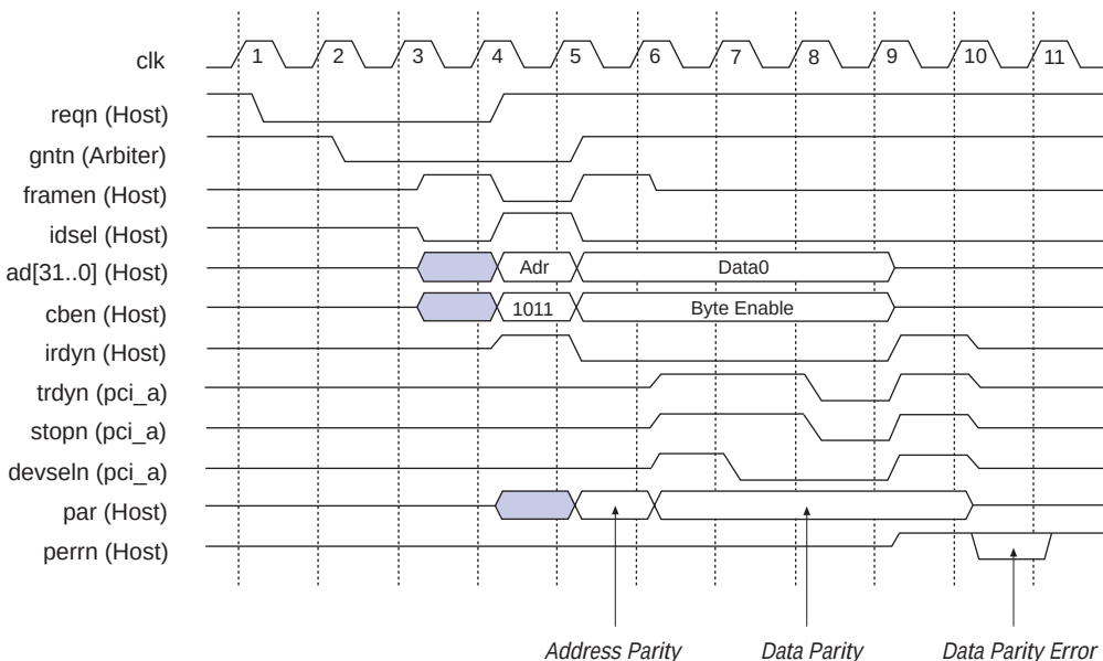
図12 コンフィギュレーション・ライト・トランザクション
