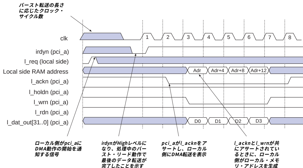
図17 PCIバスDMAリード・トランザクション
