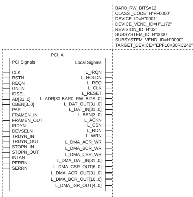
図1 pci_aのシンボル
