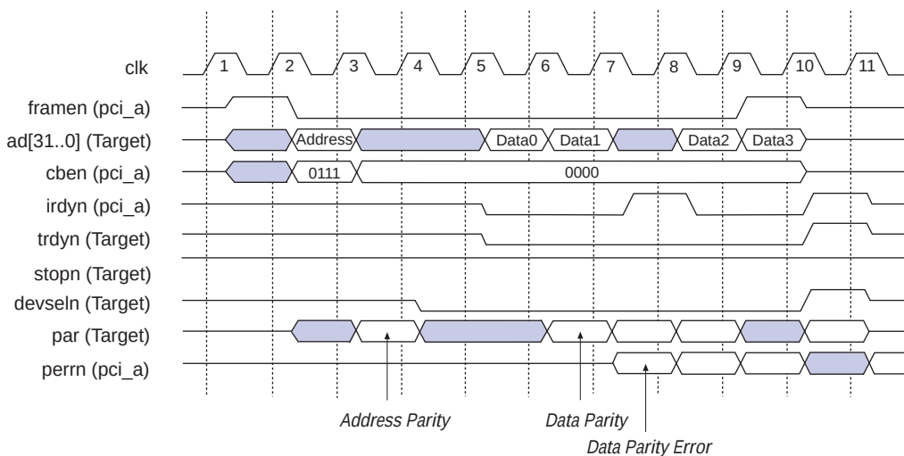
図16 マスタ・バースト・ライト・トランザクション
