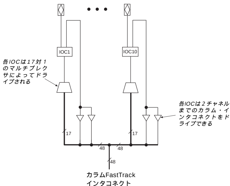
図 9 MAX 9000のカラム・インタコネクトとI/Oセルとの接続
