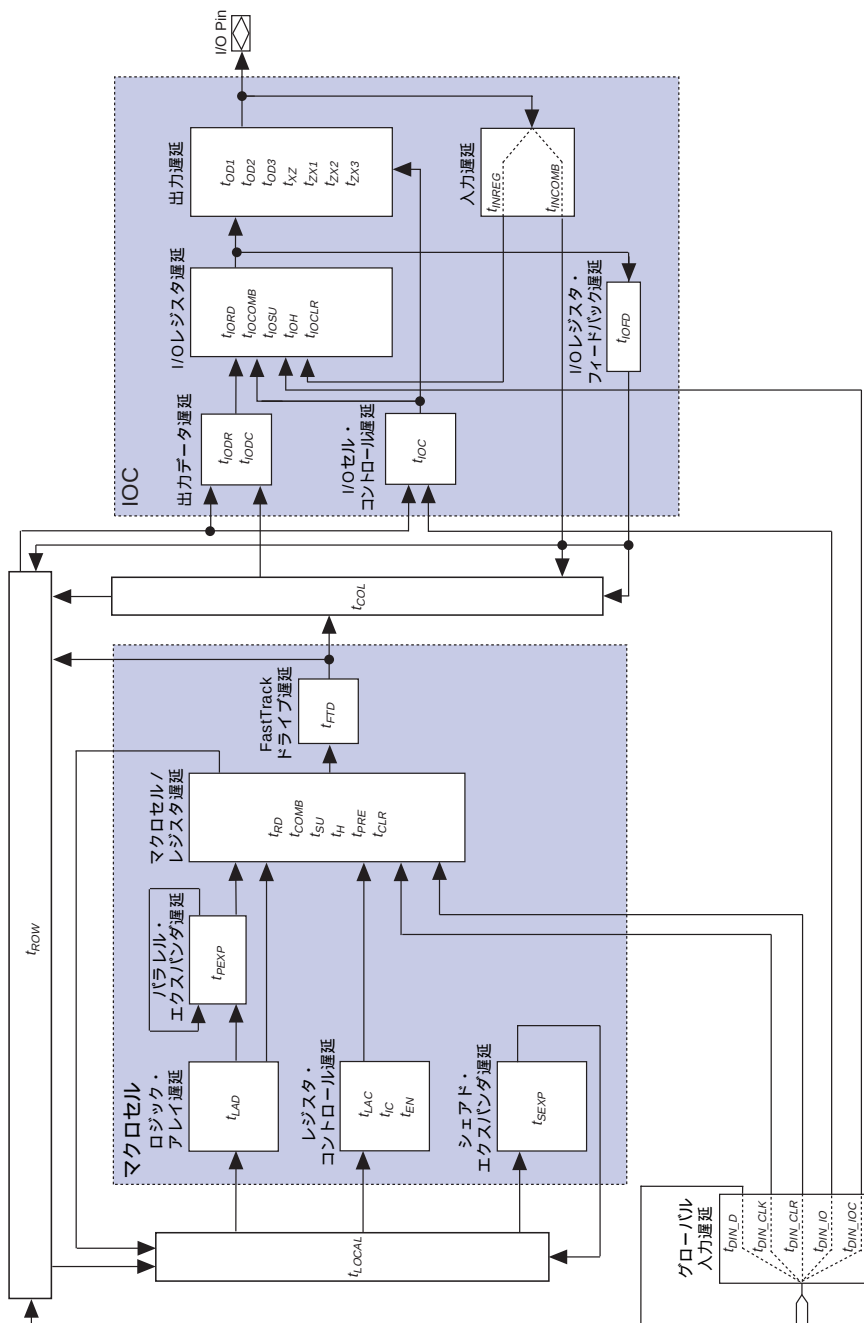
図14 MAX 9000のタイミング・モデル
