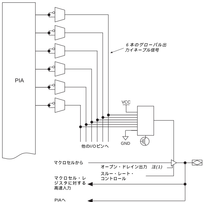
MAX 7000EとMAX 7000Sデバイス
