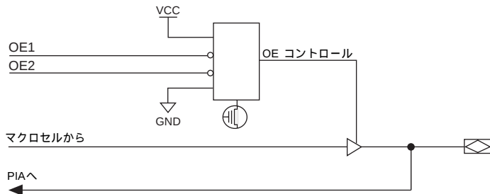
MAX 7000EとMAX 7000Sデバイス
