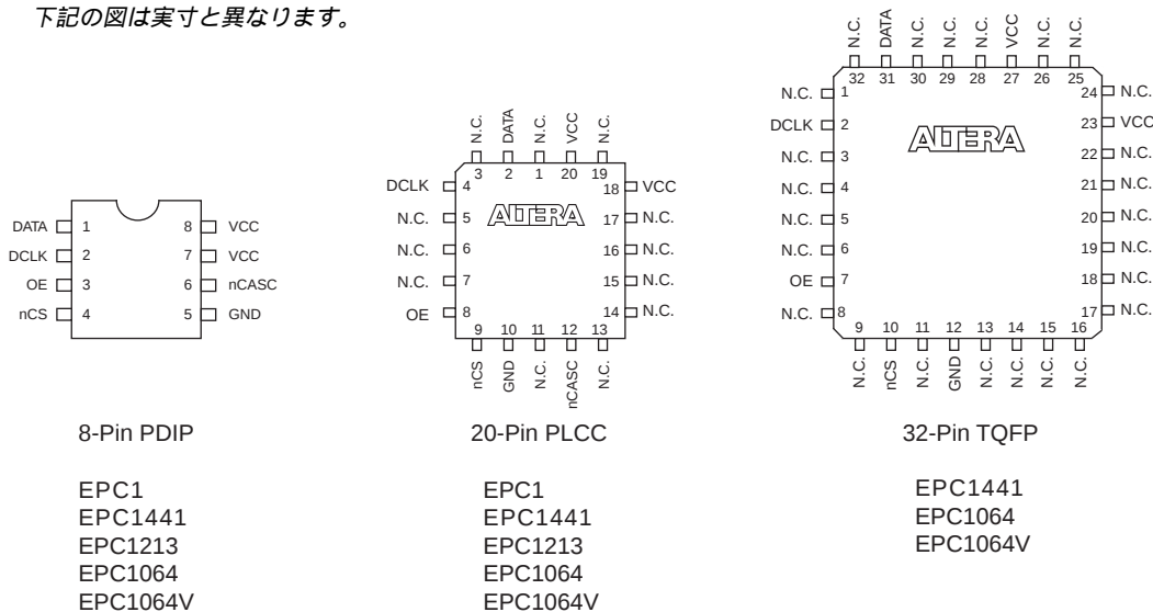
図1 コンフィギュレーションEPROMのピン配置図
